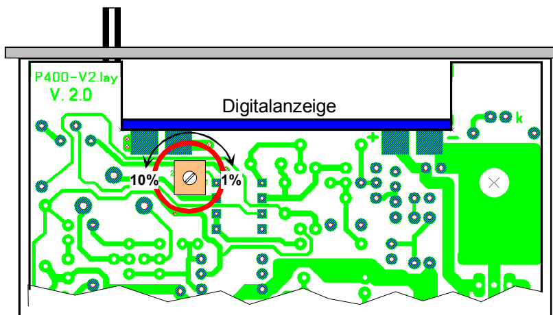
Gehäuse von unten gesehen
